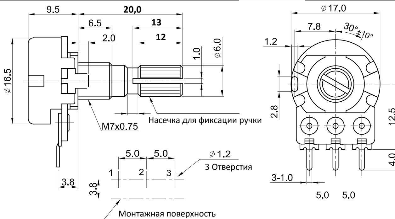
ЧЕРТЕЖ резистора 01R203 20 кОм
